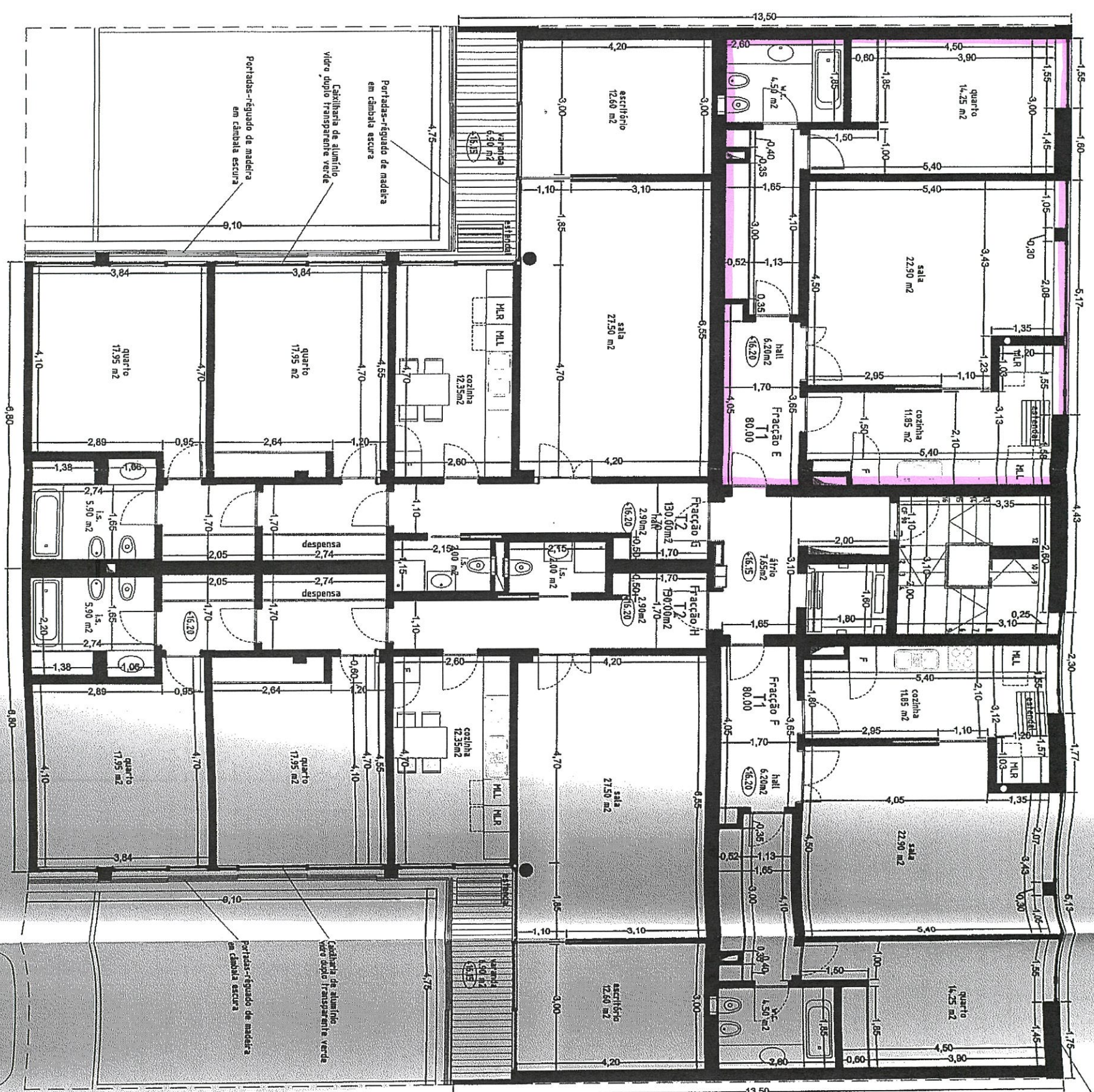
Planta Piso +1 - escala 1:100 cota +16,20
