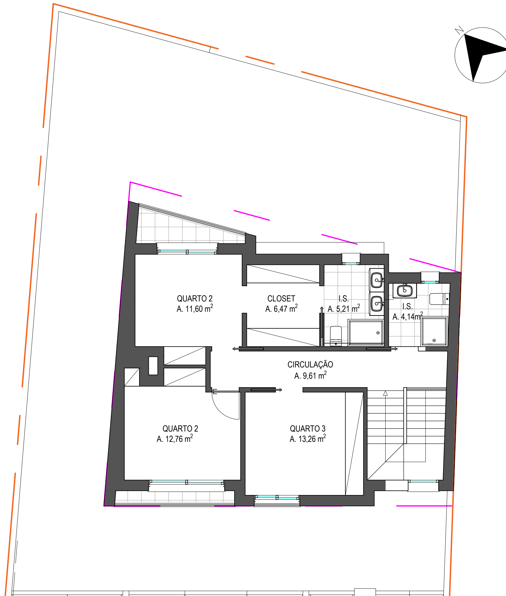
PLANTA PISO 1
