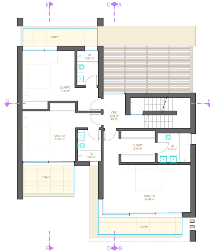
PLANTA DO 1º PISO - ÁREA: 105,06 m²
