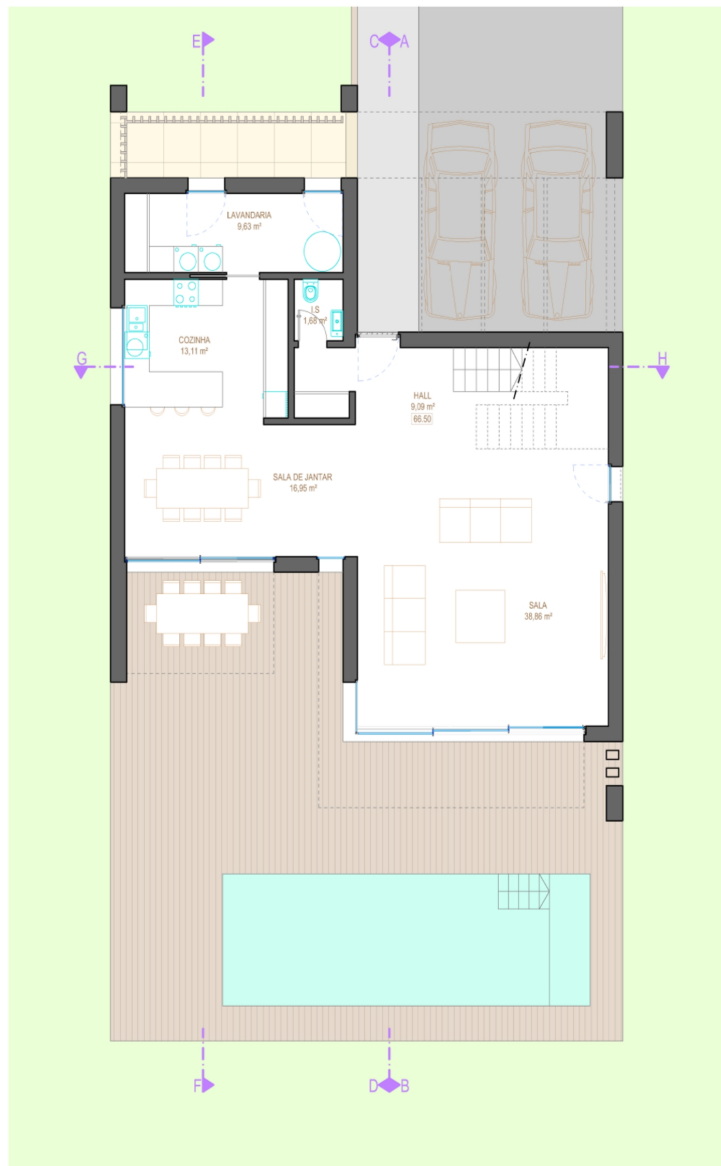
PLANTA DO PISO TÉRREO - ÁREA: 115,94 m²
