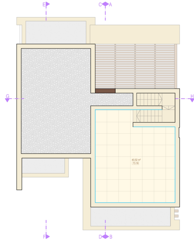
PLANTA DA COBERTURA
