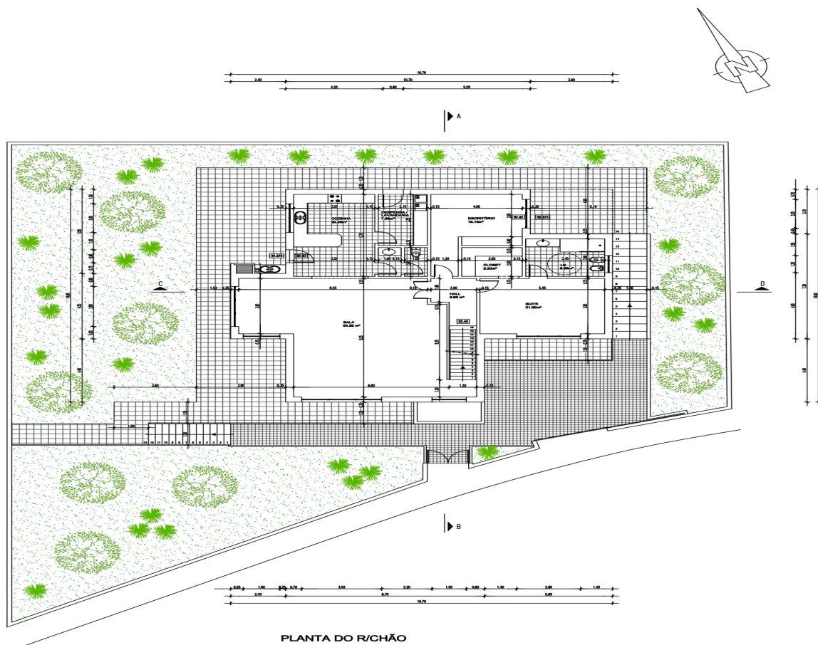
PLANTA DO R/CHÃO
