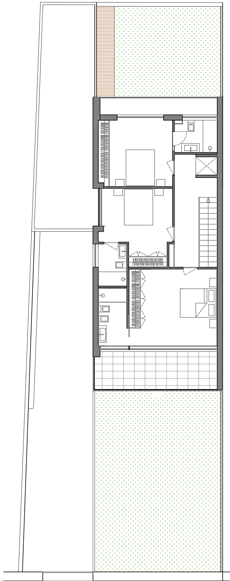
PLANTA DO PISO 01
