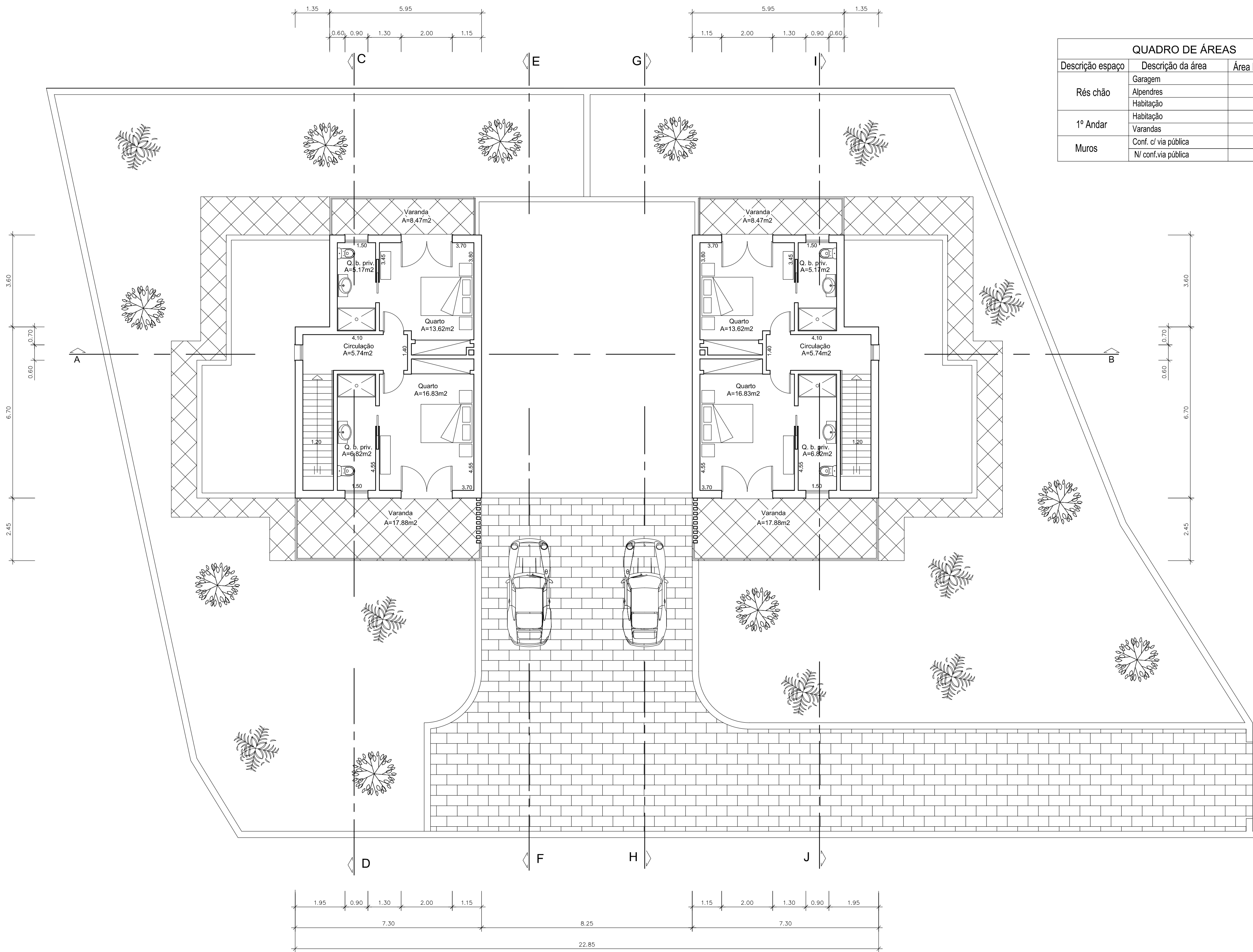
PLANTA 1º ANDAR
