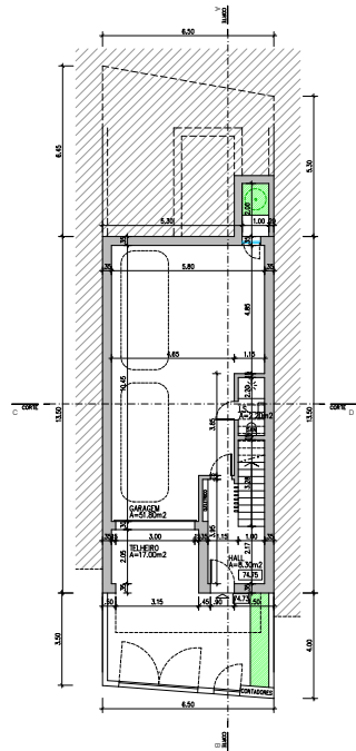
PLANTA DO PISO 0
