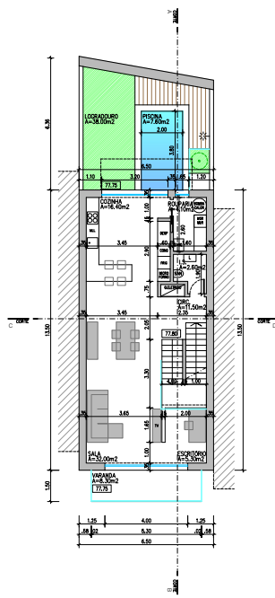
PLANTA DO PISO 1
