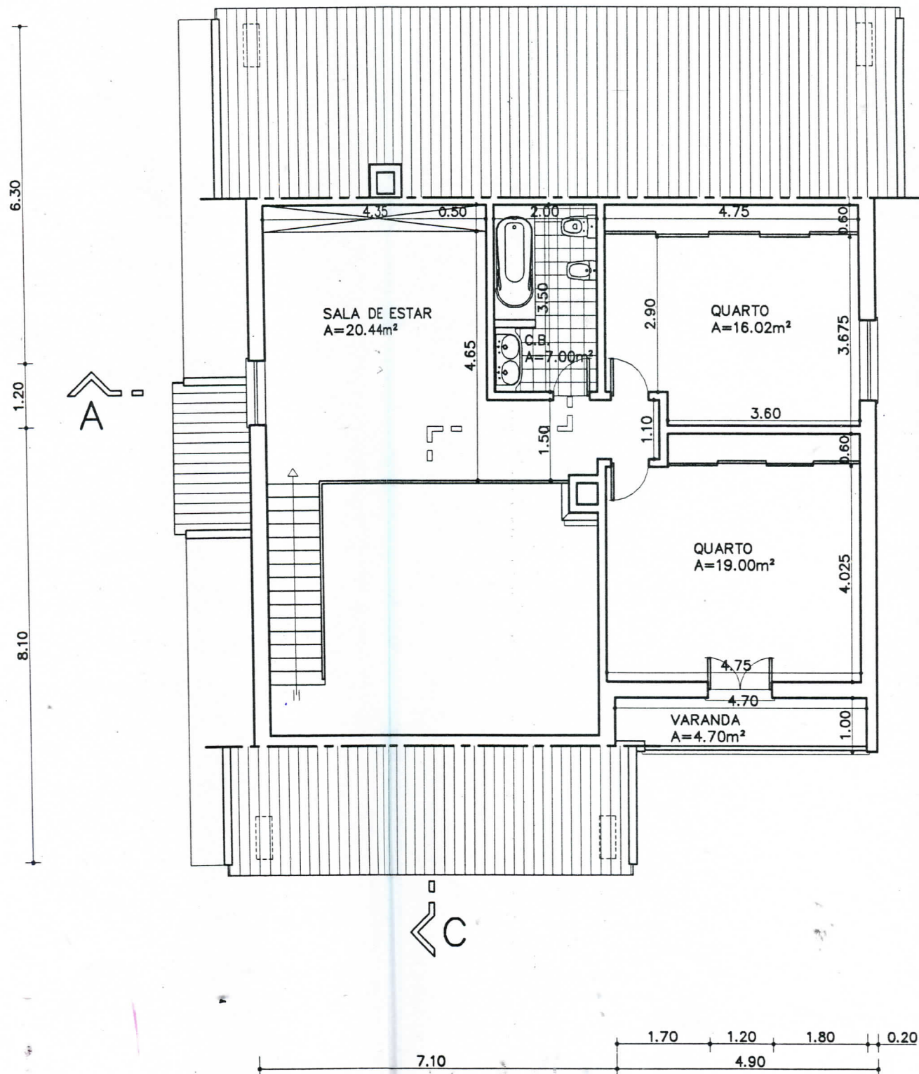
PLANTA DO 2º PISO
