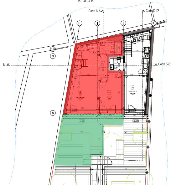
PLANTA DO PISO 0 (cota 8,23) BLOCO B
