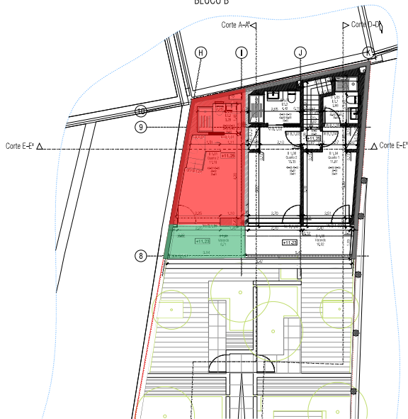
PLANTA DO PISO 1 (cota 11,23) BLOCO B
