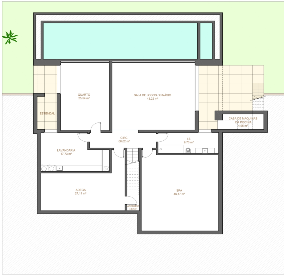
PLANTA DA CAVE - ÁREA: 219,74 m 2
