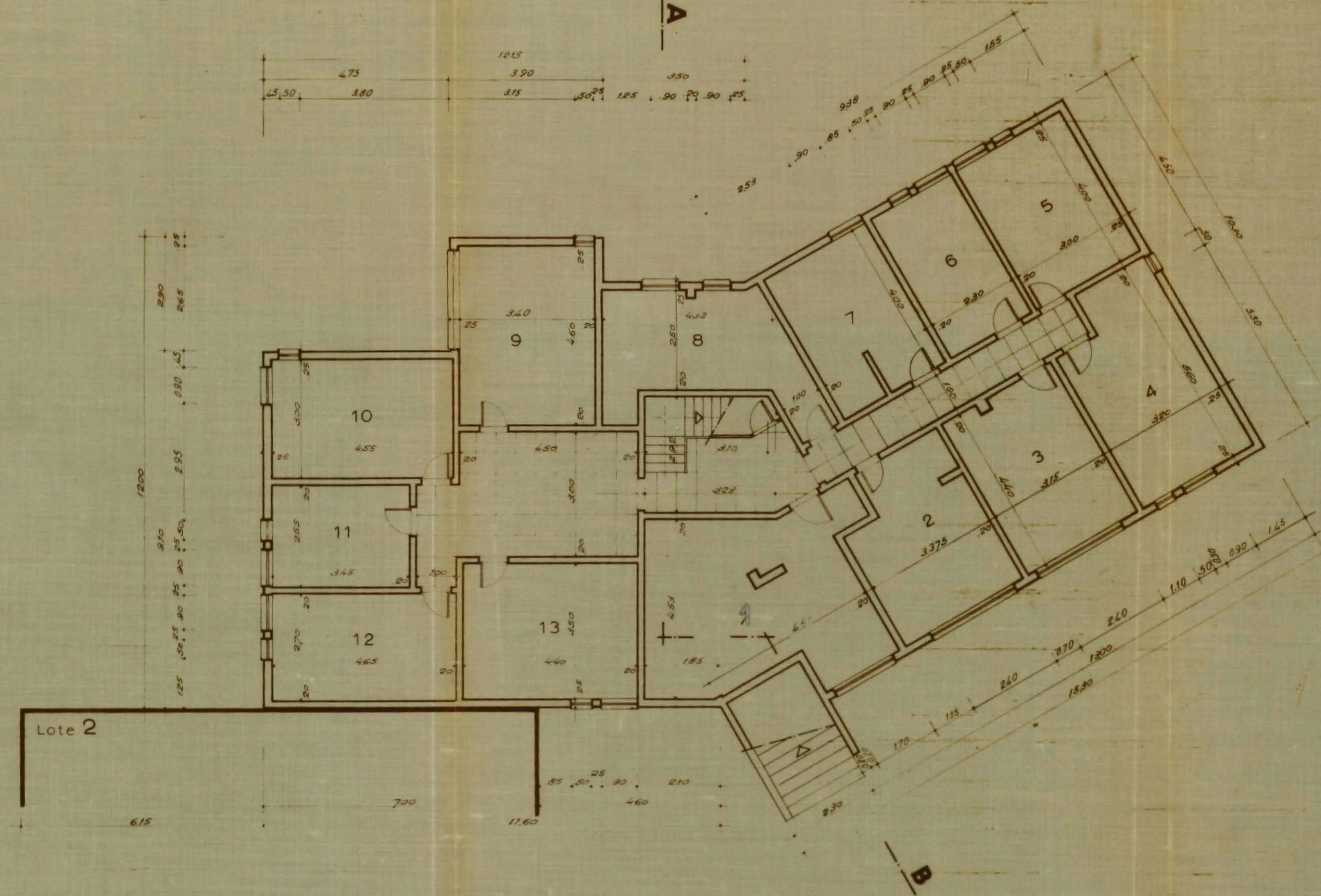
PLANTA DA CAVE (arracadações)
