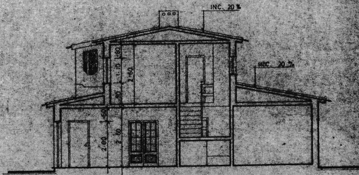
CORTE 1-1
