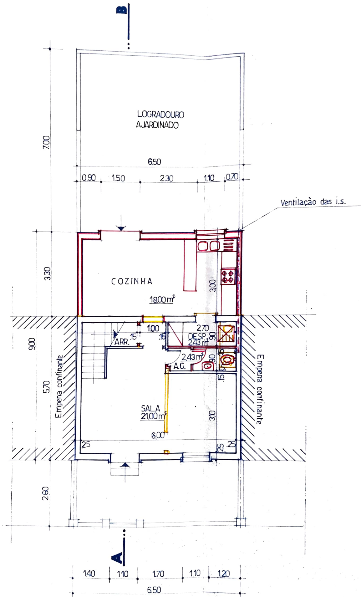
PLANTA DO RÉS-DO-CHÃO
