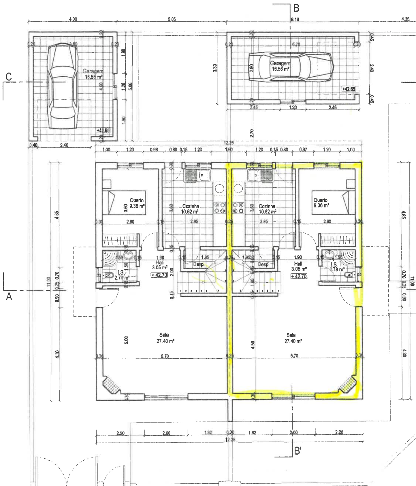
PLANTA DO RÉS-DO-CHÃO
