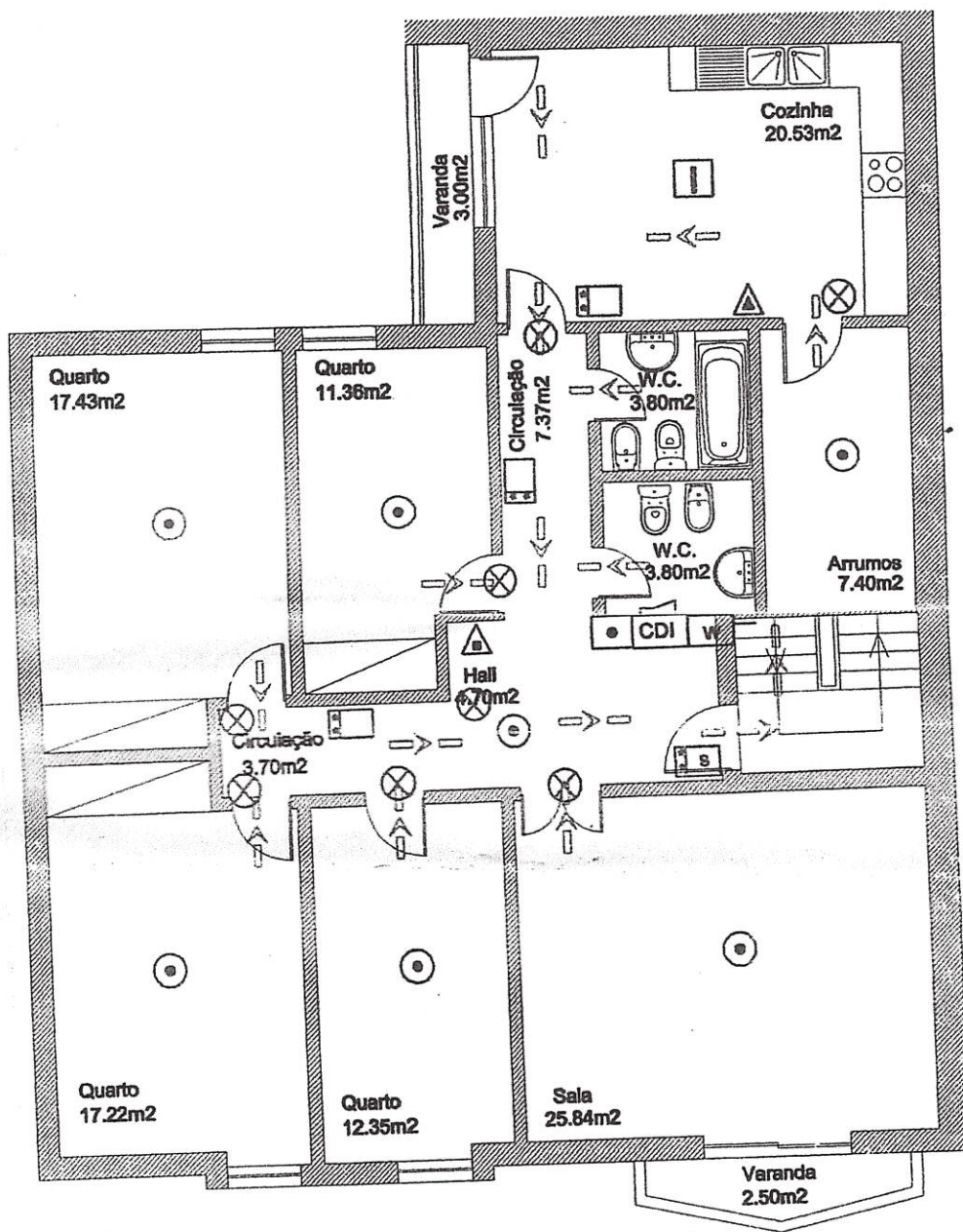
PLANTA DO 2º ANDAR
