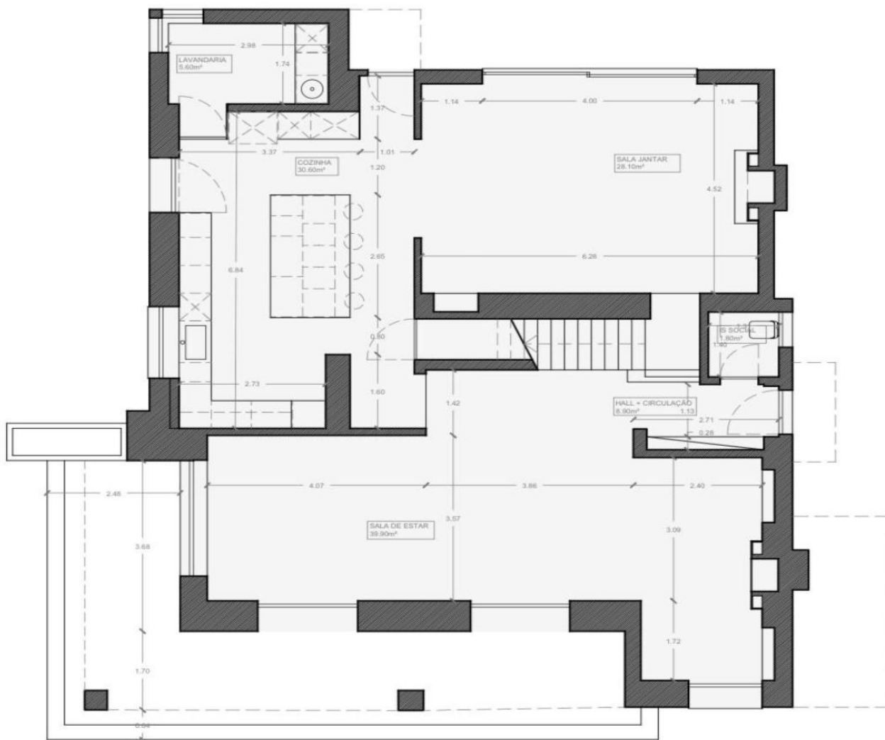
0 1 4 PLANTA GERAL - PISO 0
