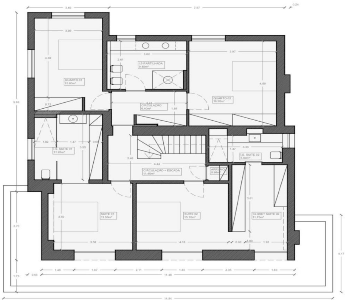
0 1 4 PLANTA GERAL - PISO 01
