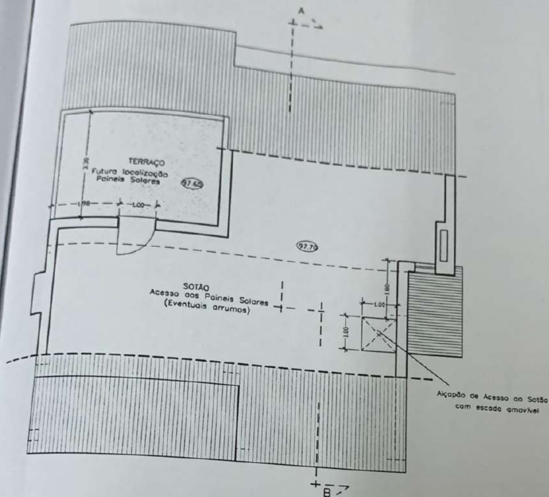
PLANTA DO SOTÃO
