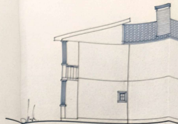
alçado lat. direito
