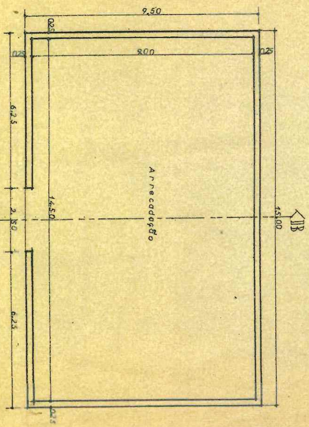
PLANTA
