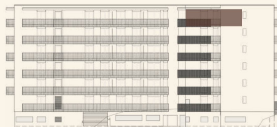
FACHADA NORTE
