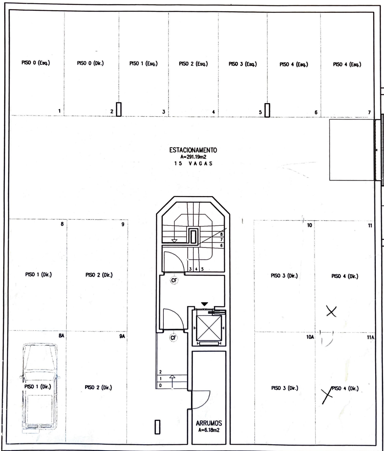
LOTE 15 PLANTA DO PARQUEAMENTO 1/100
