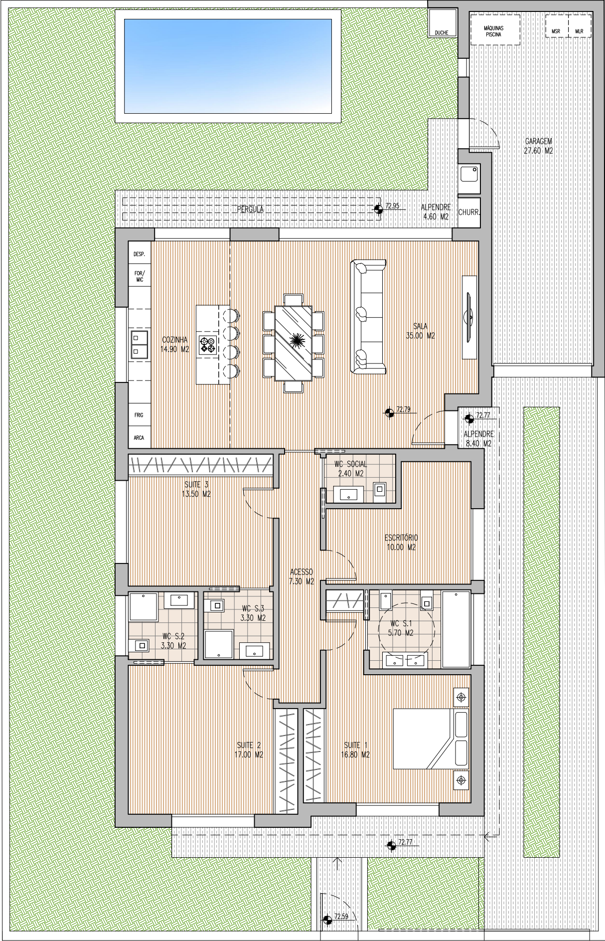
"Layout preliminar de planta de arquitetura"
