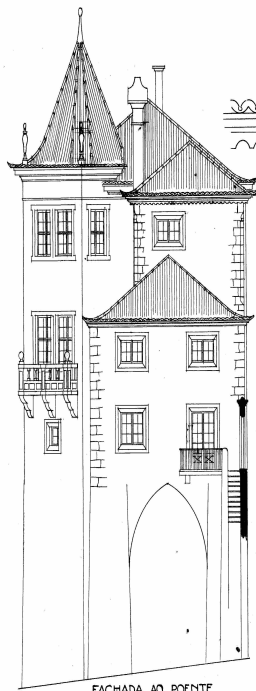
FACHADA AO POENTE
