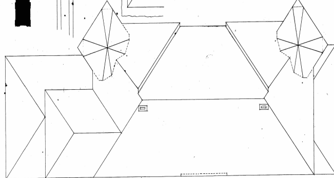
PLANTA DA COBERTURA
