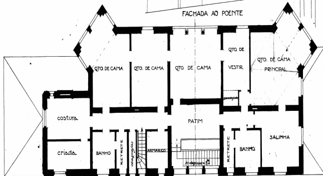
PLANTA DO PRIMEIRO ANDAR
